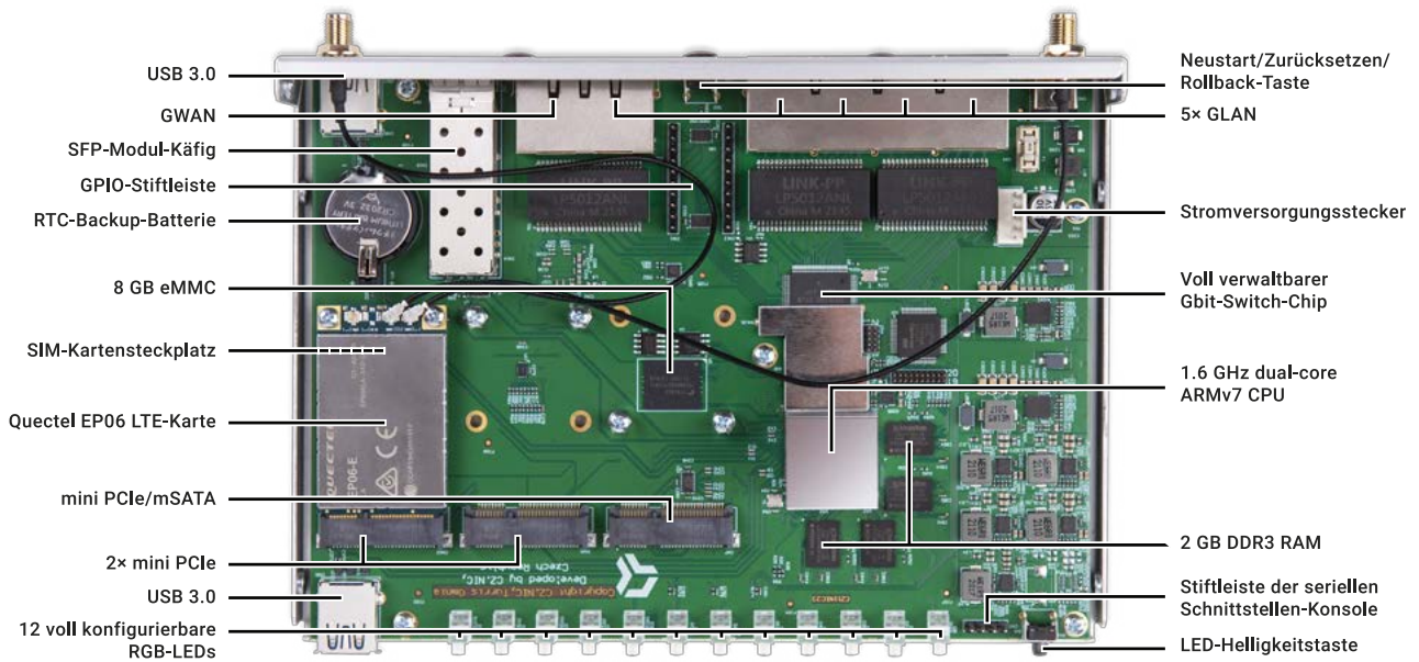
Turris Omnia 4G: Hauptplatinen-Komponenten
