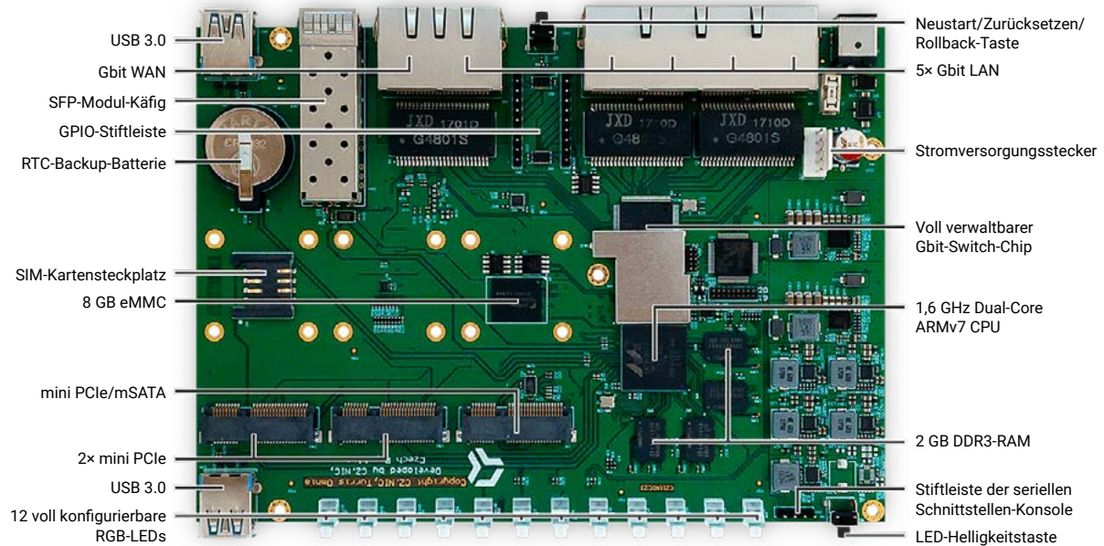
Turris Omnia No Wi-Fi: Hauptplatten-Komponenten
